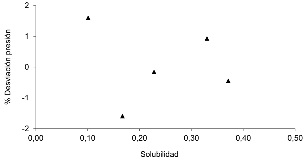
Fig. 1: Desviaciones entre los valores calculados y experimentales de la presión frente a los datos experimentales de solubilidad para el sistema N_2O + [BMIM][BF_4] a temperatura T = 293 K, utilizando el modelo PR/KM.
