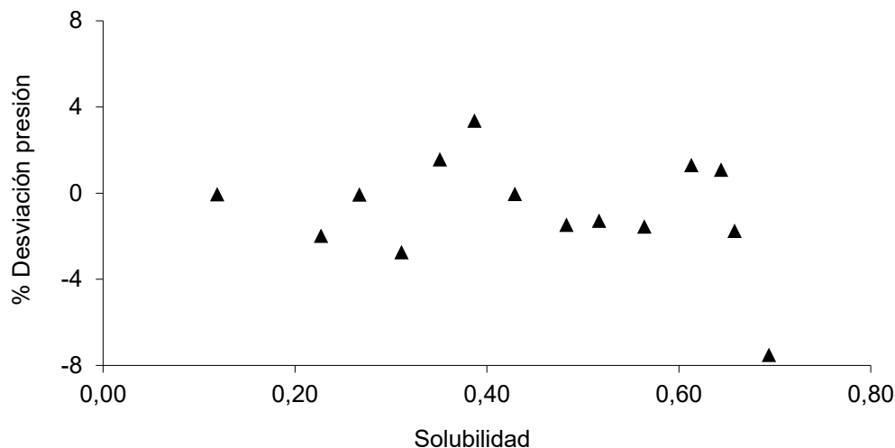
Fig. 3: Desviaciones entre los valores calculados y experimentales de la presión frente a los datos experimentales de solubilidad para el sistema \text{N}_2\text{O} + [(\text{ETO})_2\text{IM}][\text{Tf}_2\text{N}] a temperatura T = 363 K, utilizando el modelo PR/KM.
